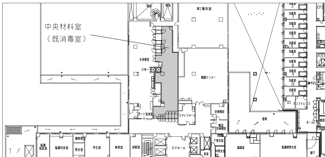
2階拡大図
